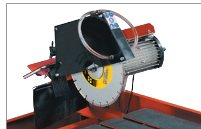
Cabezal regulable en altura para corte hasta 225 mm en 2 pasadas
